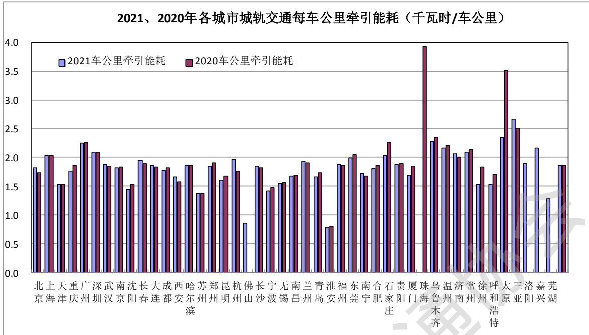
图 17 2021、2020 年各城市城轨交通每车公里牵引能耗
