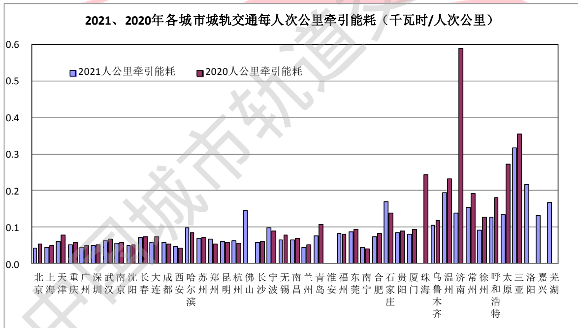
图 18 2021、2020 年各城市城轨交通每人公里牵引能耗
